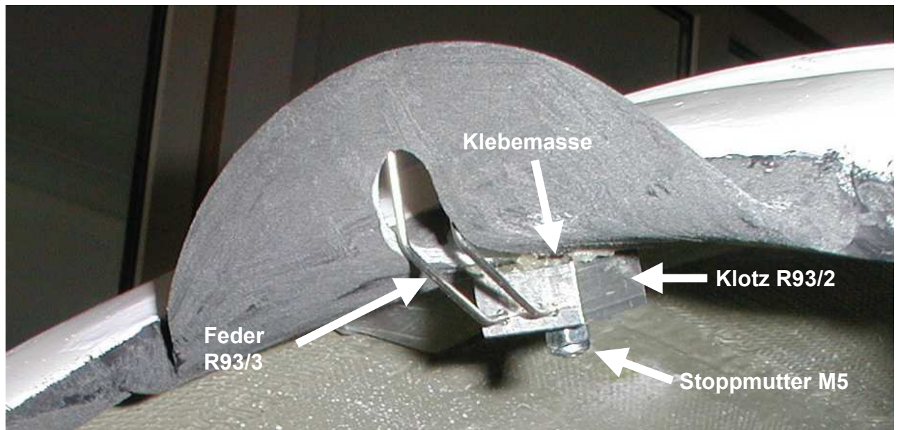
Abbildung 5: Fertig montierte Führung von unten
