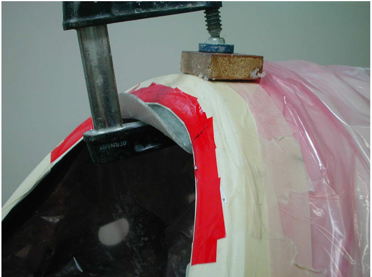
Abbildung 3: Verklebung
